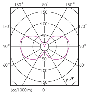
LEDBulb E27 400lm
