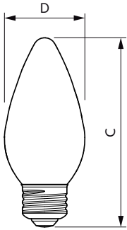
Candle F15 60W 500lm 2700-2200K E26 D CL
