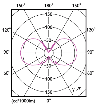
LEDbulb CLA F15 5,5W E26 922 927 CL-LDD
